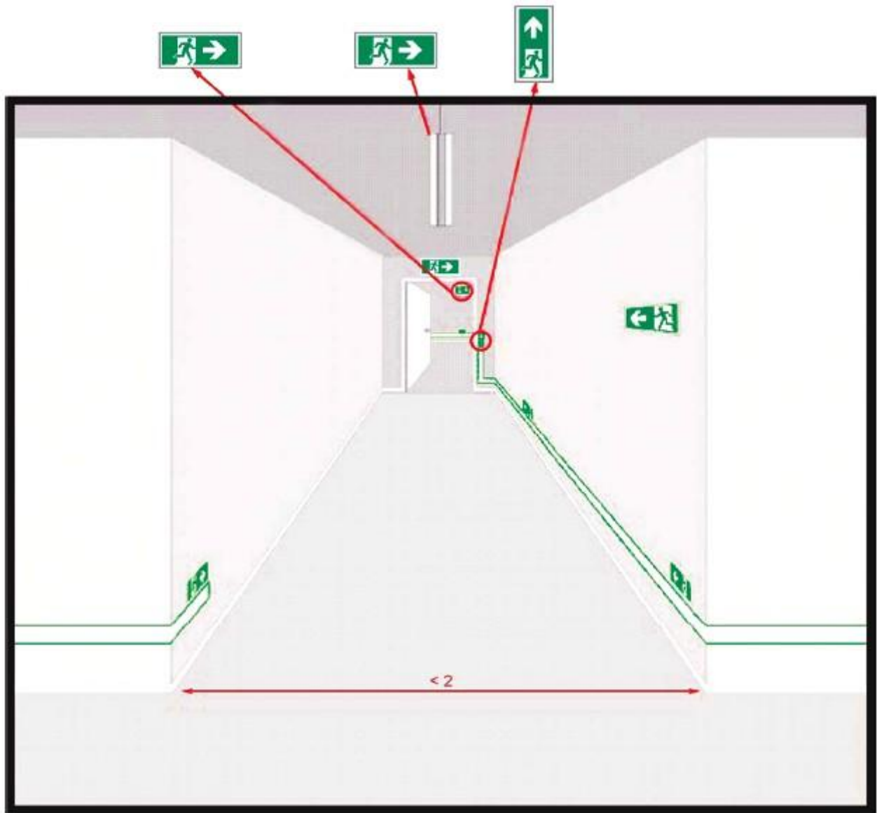
Рисунок А.1 - Примерный план Т-образного перекрестка, ведущего в прямой коридор шириной не более 2 м и длиной не более 10 м
